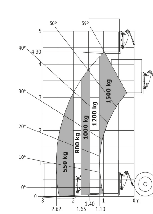
Rough terrain load chart (EN1459 B) 500 mm load center
